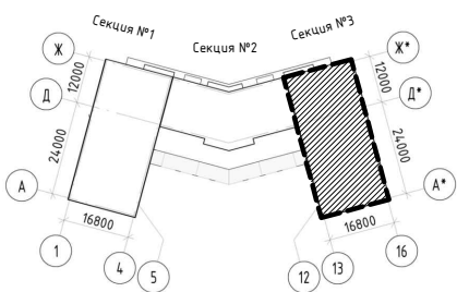
Компновочная схема
